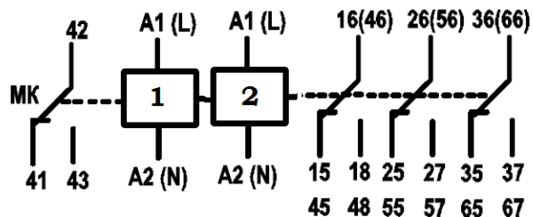
Рис 3. Диаграмма работы реле.
